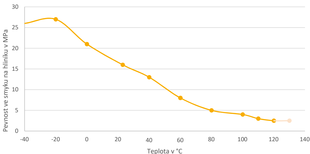
Pevnost ve smyku na hliníku v závislosti na teplotě
